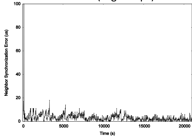
GTSP (avg: 2.8 \mu\text{s} )
