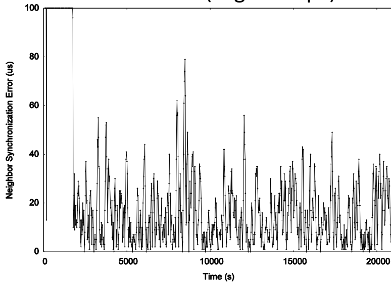
FTSP (avg: 15.0 \mu\text{s} )
